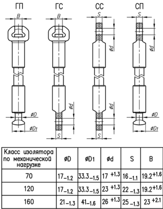
Исполнения изоляторов по типам применяемых оконцевателей
