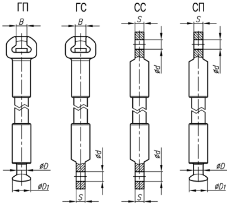
Исполнения изоляторов по типам применяемых оконцевателей
